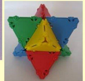
звездчатый тетраэдр
