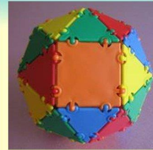
курносый куб
